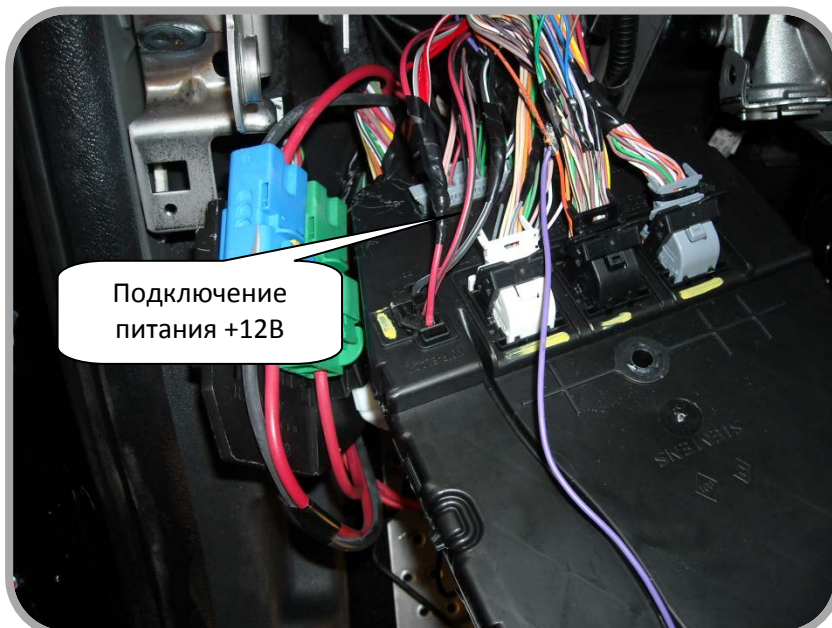
Рисунок 6 – Подключение питания +АКБ
