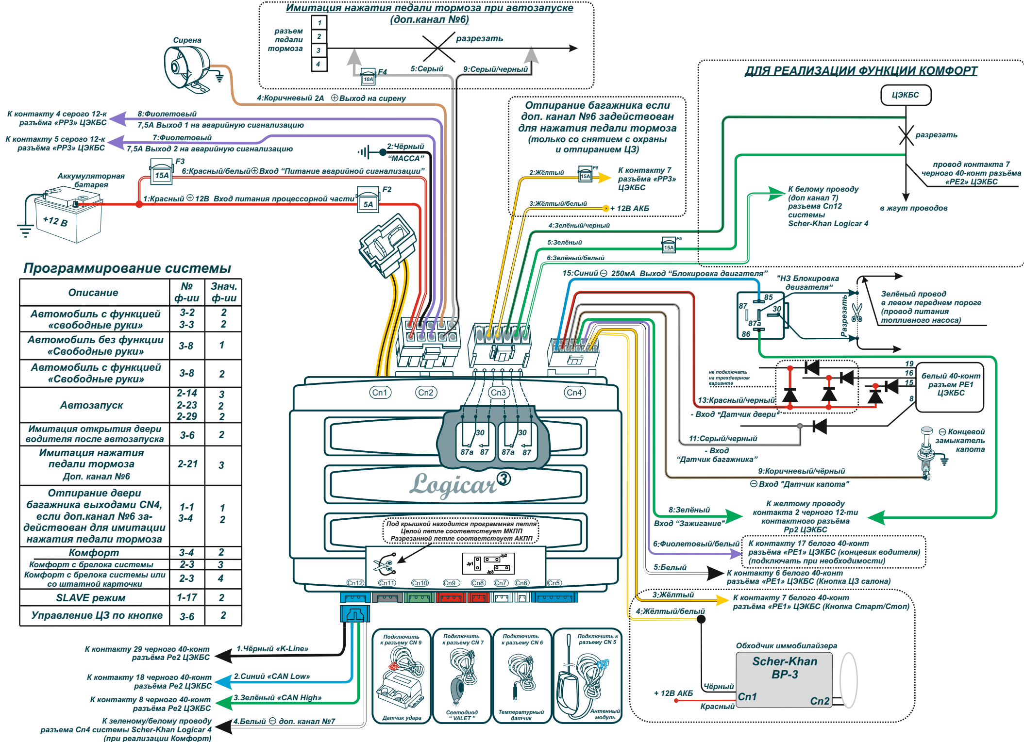
Схема подключения системы Scher-Khan Logicar 3 к автомобилю Renault Clio 3 (карточка)
