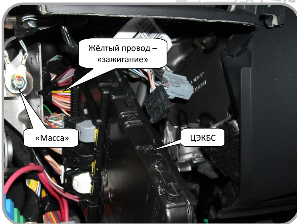
Рисунок 2 - Подключение датчика зажигания.
