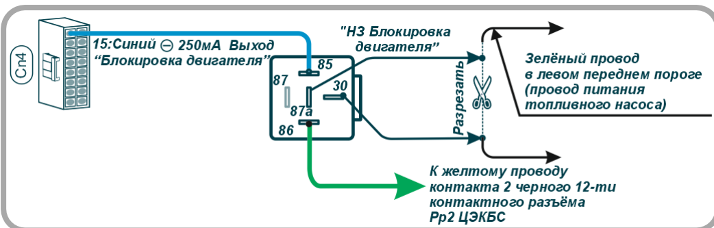
Схема 3 – Подключение цепи блокировки
