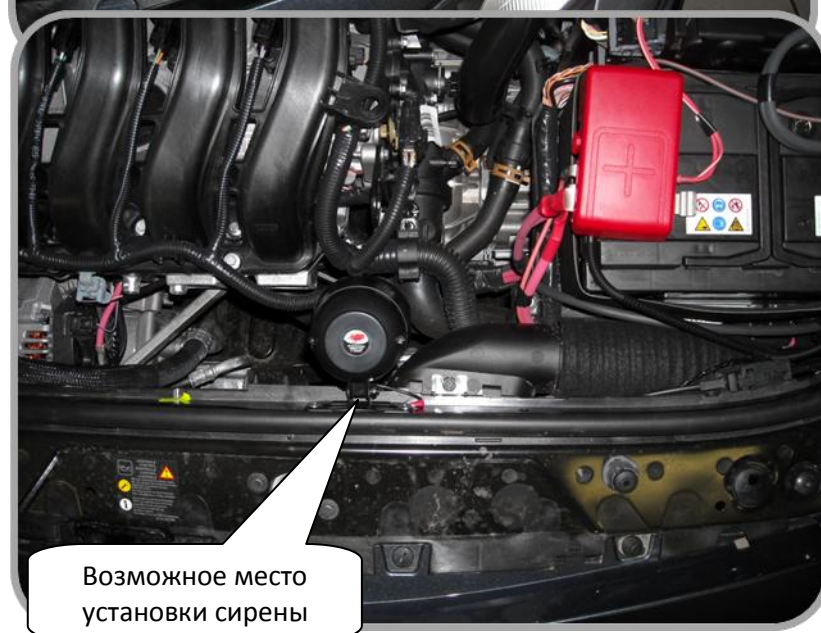
Рисунок 5 – Возможное место установки сирены
