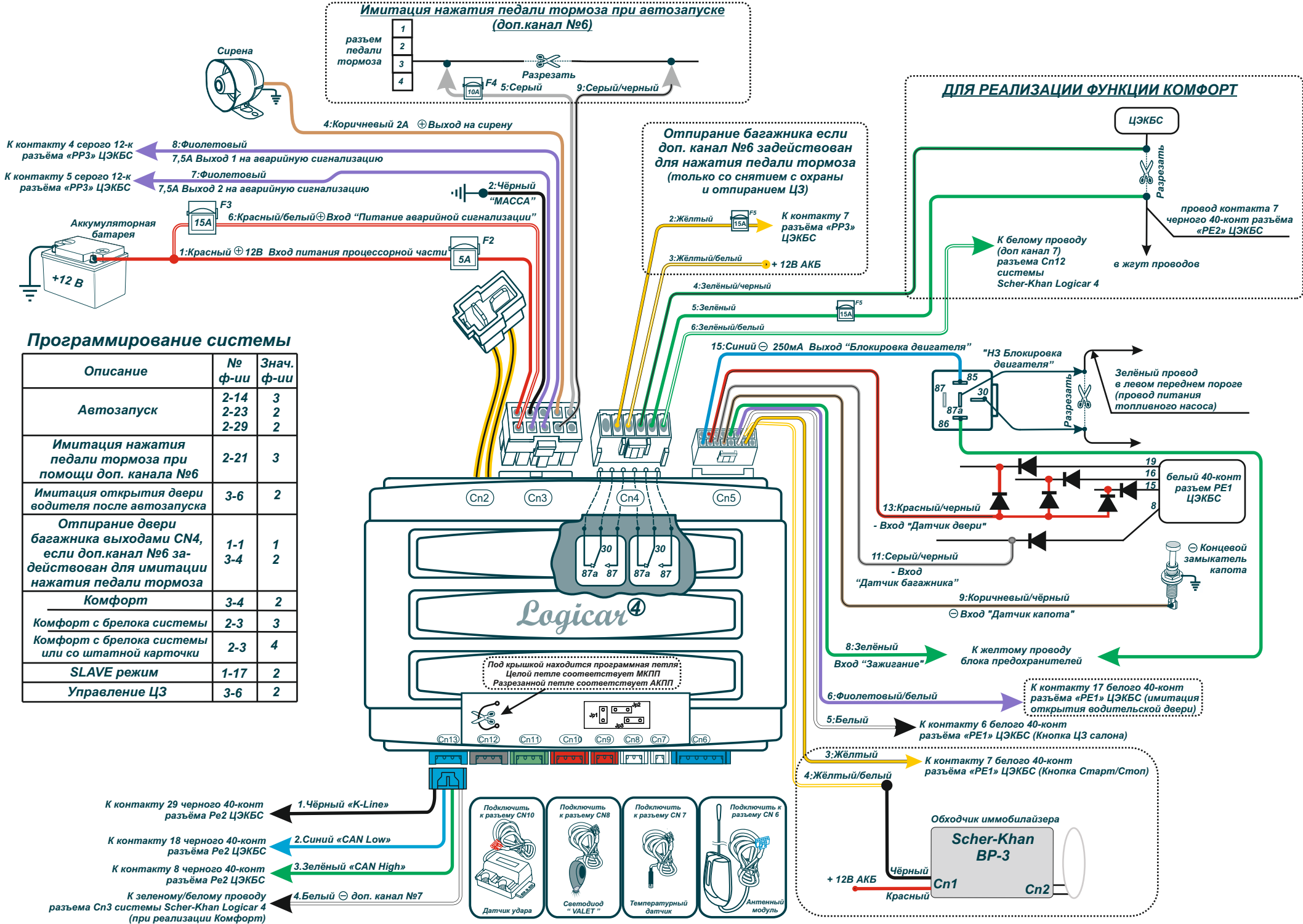
Схема подключения системы Scher-Khan Logicar 4 к автомобилю Renault Megane II
