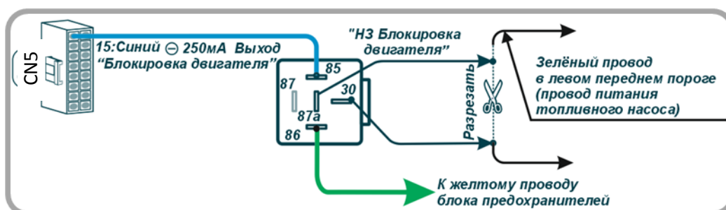
Схема 3 – Подключение цепи блокировки
